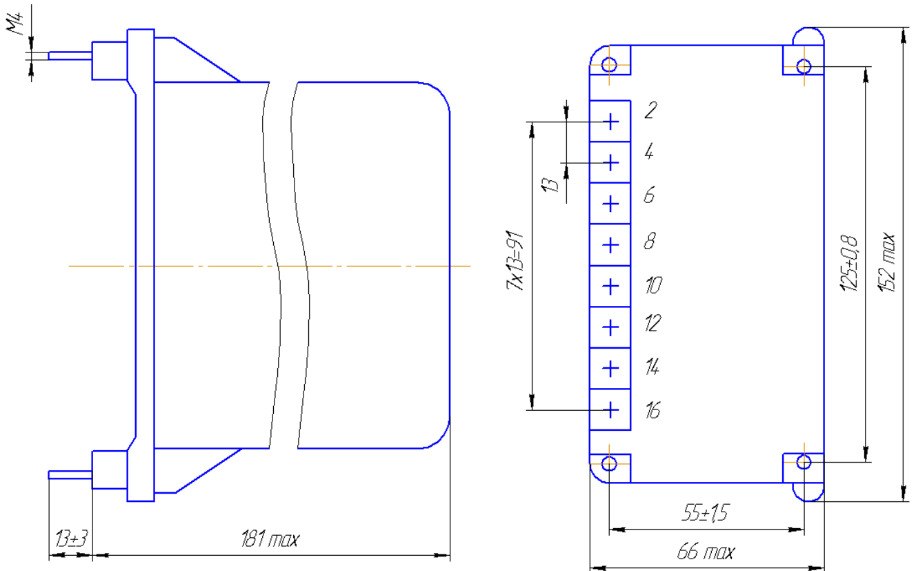
Рисунок 1 – Габаритные, установочные, присоединительные размеры реле РСТ11М.
